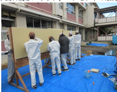
ボード開口及びスイッチ、コンセントの取付作業
